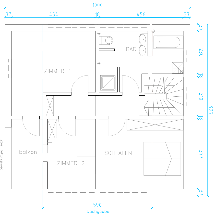
OBERGESCHOSS
