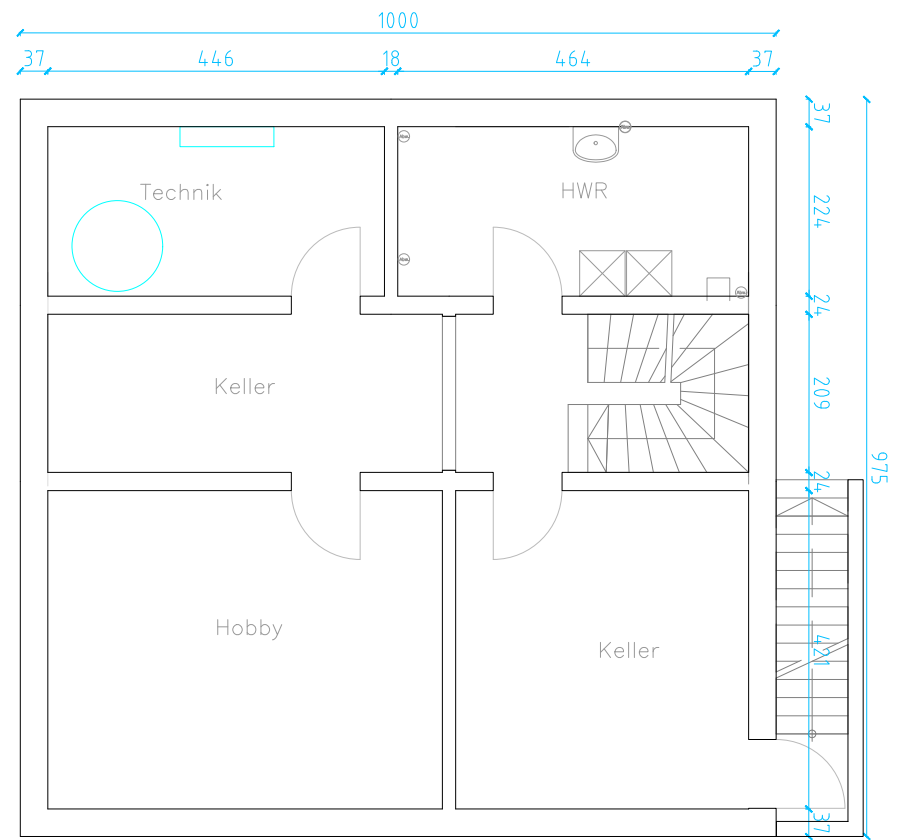
UNTERGESCHOSS
